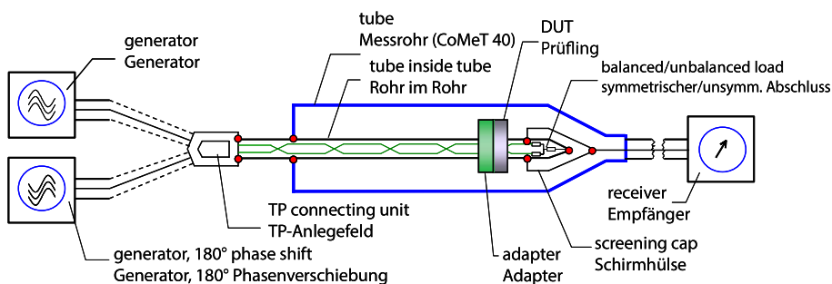
IEC 62153-4-7 Ed.3 (draft): Coupling Attenuation a_C of a Balanced Connector Kopplungsdämpfung a_C eines symmetrischen Steckers
