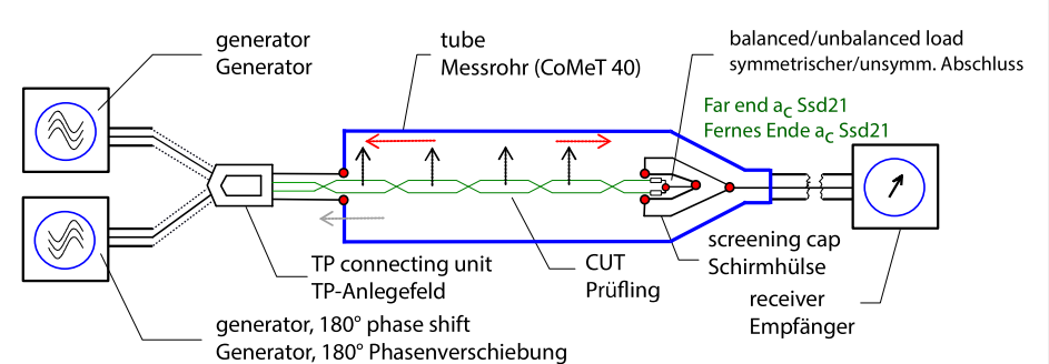
IEC 62153-4-9 Ed.2 Amd.1: Coupling Attenuation a_C of Unscreened Balanced Pairs, Far End Kopplungsdämpfung a_C ungeschirmter Paare, Fernes Ende
