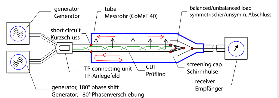
IEC 62153-4-9 Ed.2: Coupling Attenuation a_C – Triaxial Method Kopplungsdämpfung a_C – Triaxialverfahren
