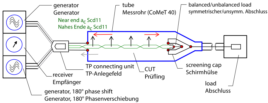
IEC 62153-4-9 Ed.2 Amd.1: Coupling Attenuation a_C of Unscreened Balanced Pairs, Near End Kopplungsdämpfung a_C ungeschirmter Paare, Nahes Ende
