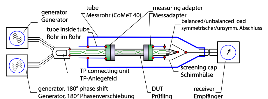
IEC 62153-4-7 Ed.3 (draft): Coupling Attenuation a_C of a Balanced Assembly Kopplungsdämpfung a_C eines symm. Assemblies
